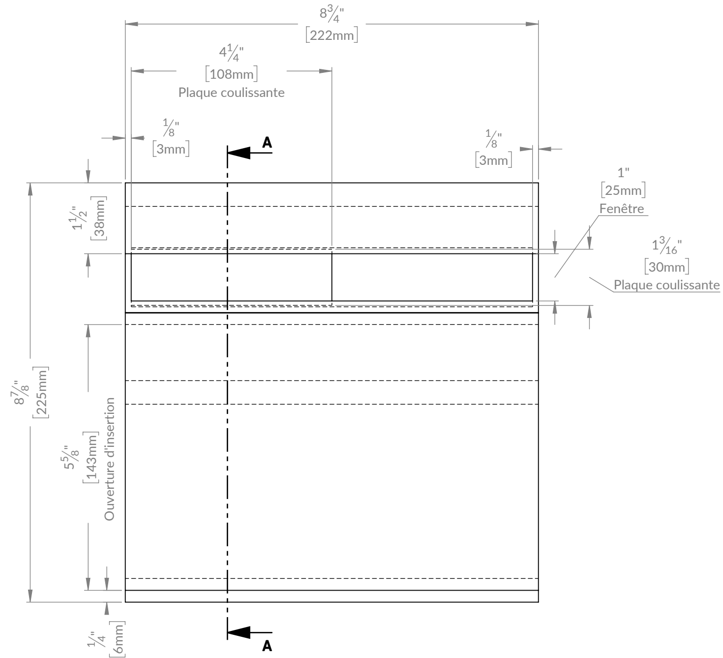
ÉLÉVATION
