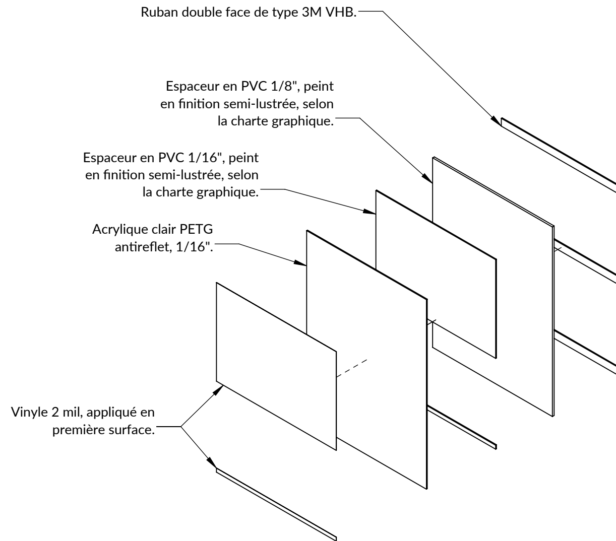
ISOMÉTRIQUE ÉCLATÉE
